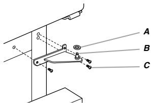
A. Shim B. Center Hinge C. Hinge Screws
